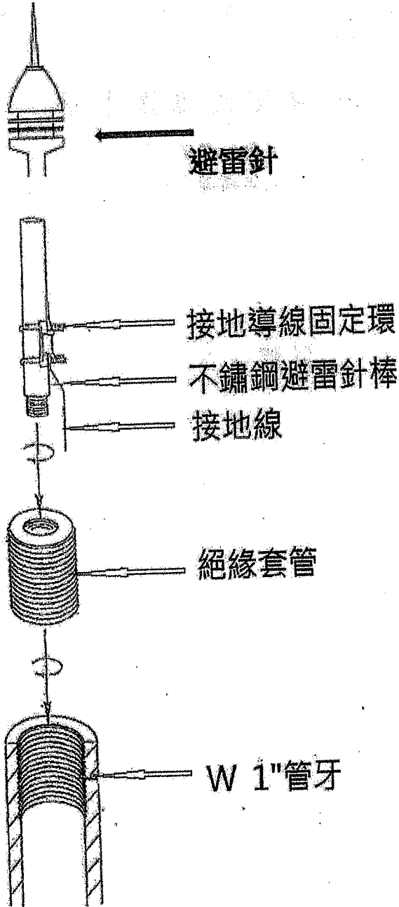
設備(避雷針)本身組裝圖
